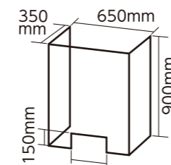
●セット内容 350mm パネル(650×900×2mm) ... 1 パネル(350×900×2mm) ... 2 コーナー用固定パーツ(材質/PVC) ... 12
