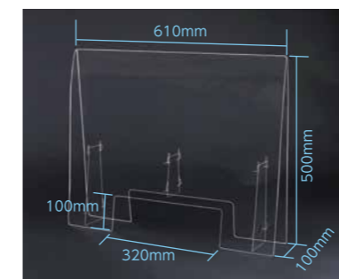
●サイズ/610×500×100mm(組立時) ●材質/PET
